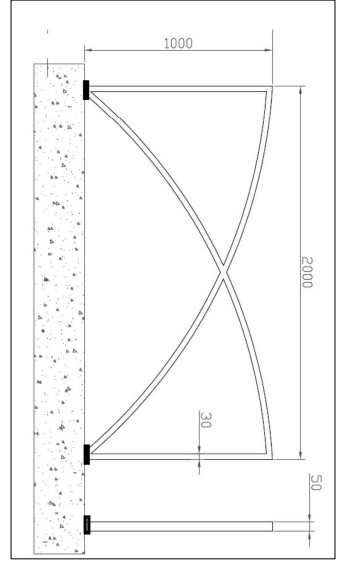
Transenna in acciaio
